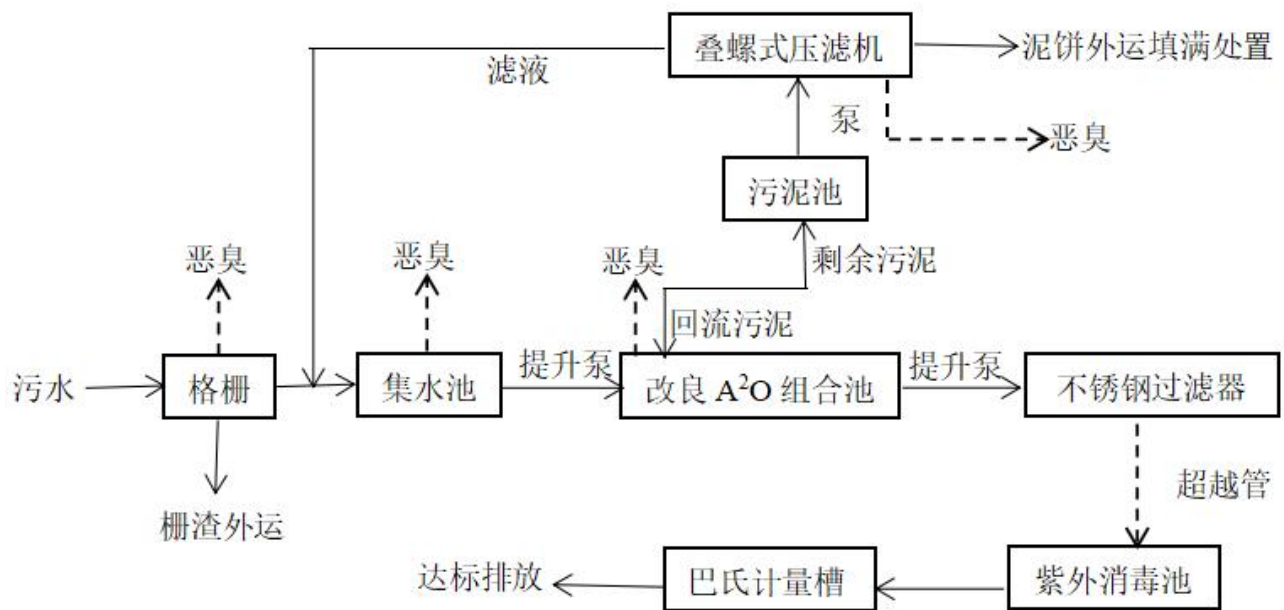
图 3-1 废水监测示意图
